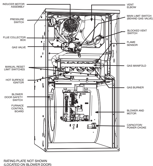
Fig. 1 – 80% AFUE Single Stage Furnace Components
