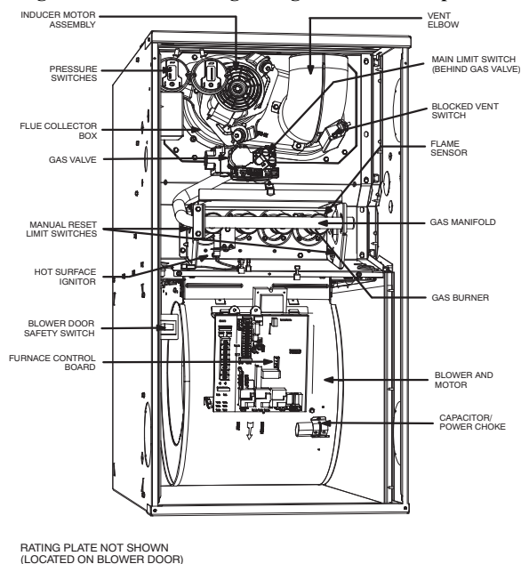
Fig. 2 – 80% AFUE Two-Stage Furnace Components
